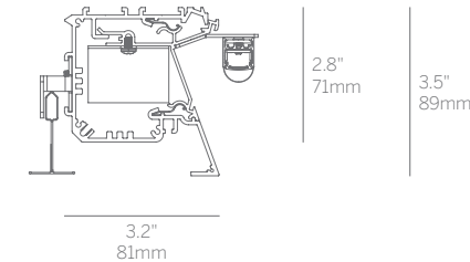
Bezel Trim (RBT)
