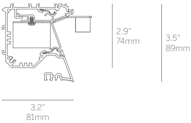
Bezel Trim
