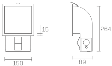
Bezel
