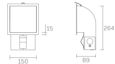
Bezel
