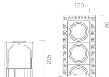
bezel
